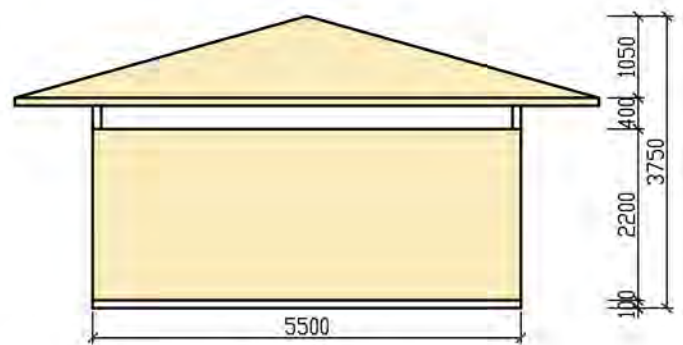
RIGHT ELEVATION
