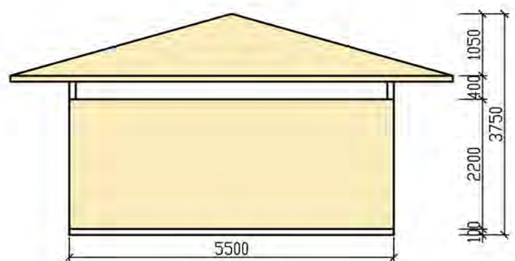
RIGHT ELEVATION
